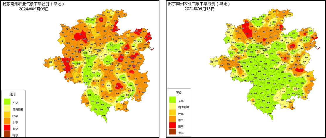
附图 2024 年 9 月 6 日（左）和 13 日（右）黔东南州农业气象干旱监测
